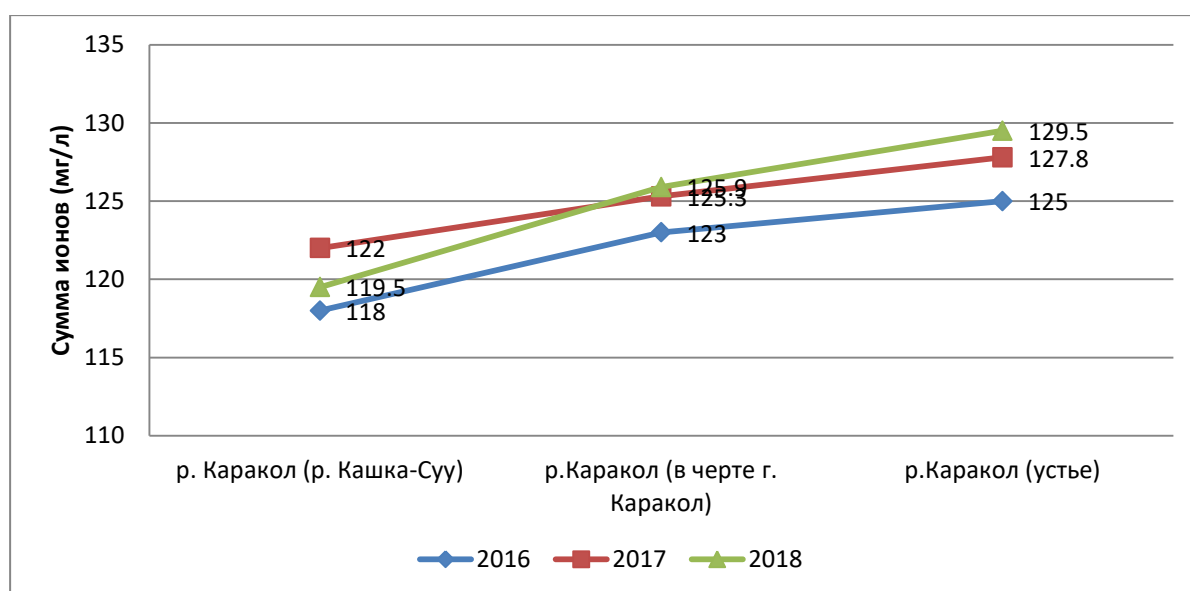
Рис. 3.1.1. Суммарное содержание ионов в воде реки.
