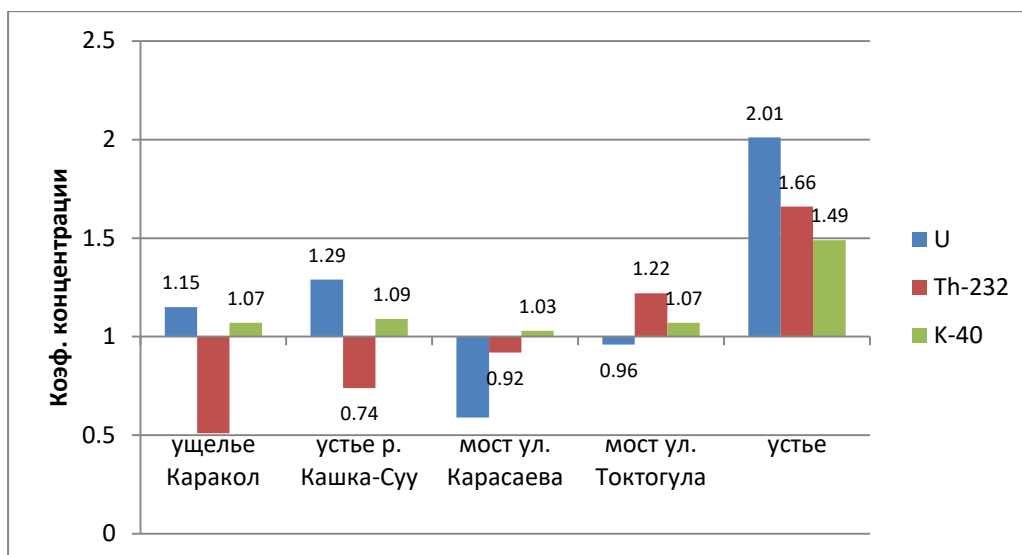
Рис. 3.1.5. Коэффициент концентрации радионуклидов в донных отложениях реки Каракол.
