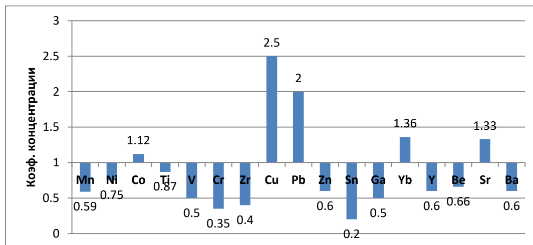
Рис. 3.1.3. Коэффициент концентрации химических элементов в донных отложениях реки Каракол в черте города.
