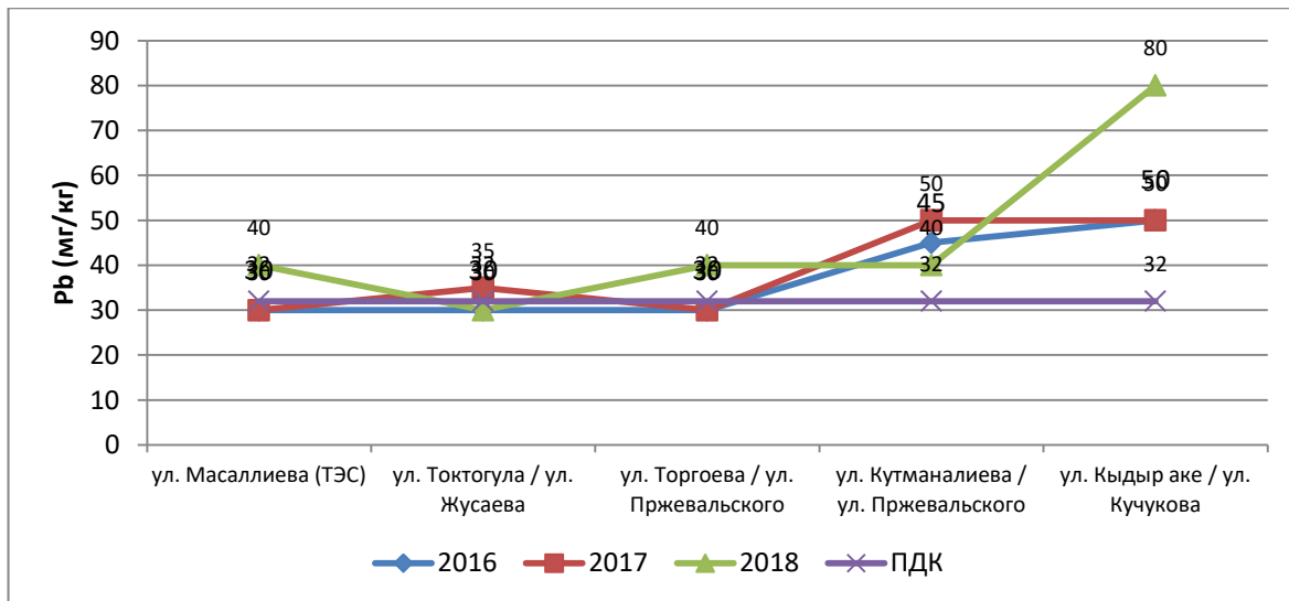
Рис. 3.2.1. Содержание свинца в отдельных зонах г. Каракол.
