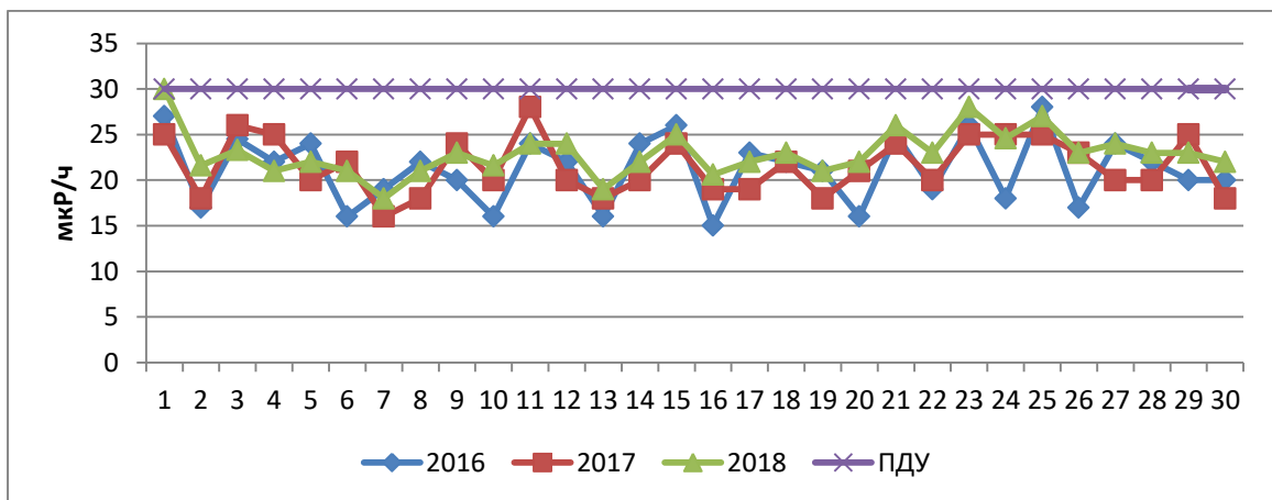
Рис. 3.6.2. Вариации уровня экспозиционной дозы на территории г. Каракол по 30 точкам измерений за 2016,2017,2018 годы.
