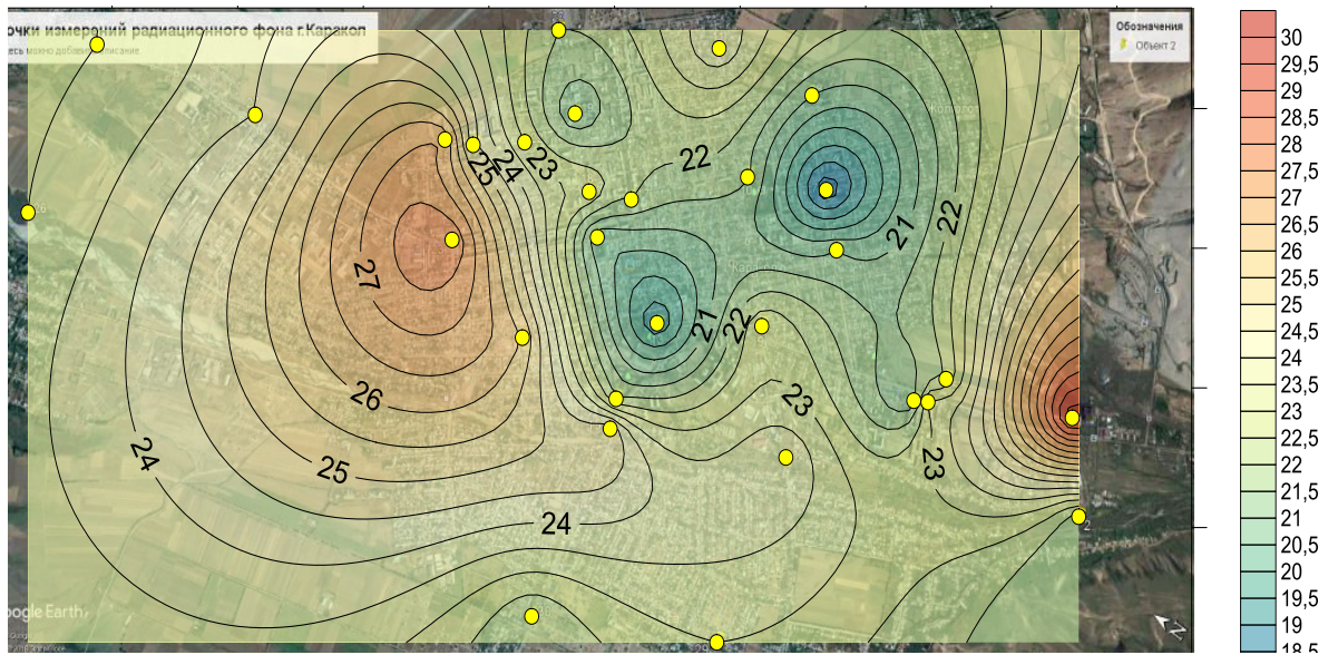
Рис. 3.6.1. Картосхема мощности экспозиционной дозы гамма-излучения на территории г. Каракол (мкР/ч).
