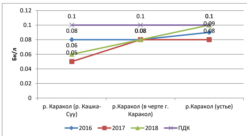
Рис. 3.1.4. Суммарная \alpha -активность воды реки Каракол за 2016, 2017, 2018 годы (март).
