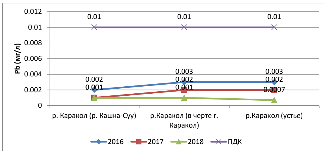
Рис. 3.1.2. Содержание свинца в воде реки Каракол.
